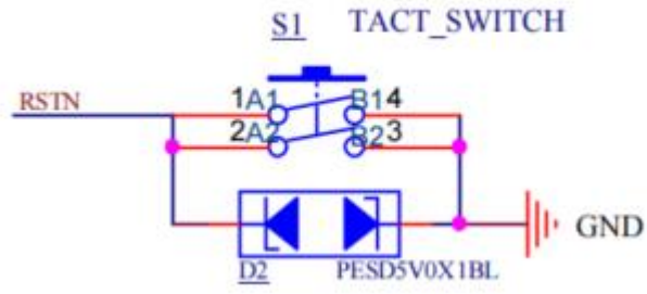
Figure 11. QD302 Reset circuit diagram / QD302复位电路示意图
