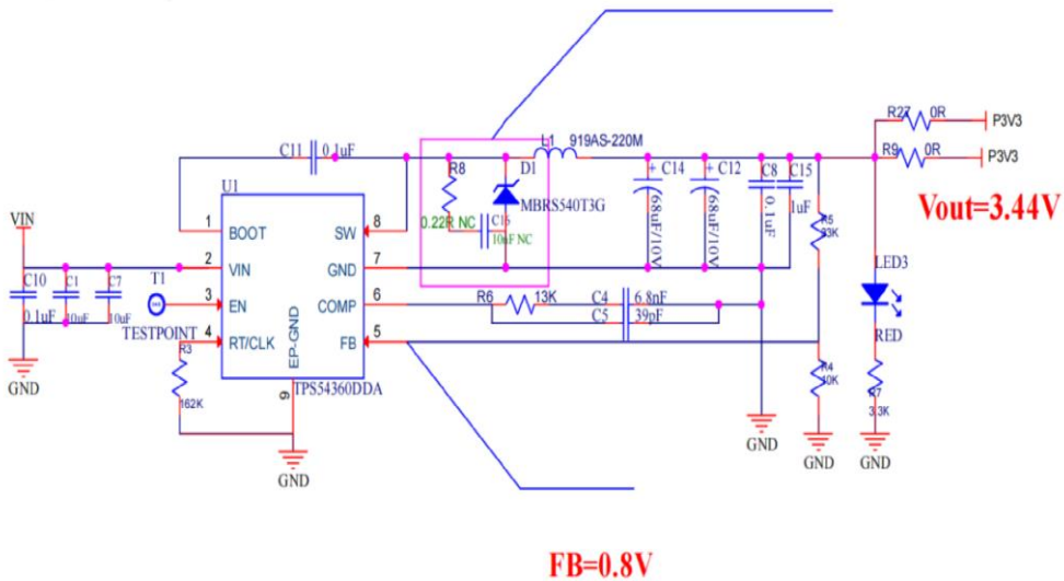
Figure 8. QD302 Power Supply Design Circuit Diagram / QD302供电设计电路示意图
