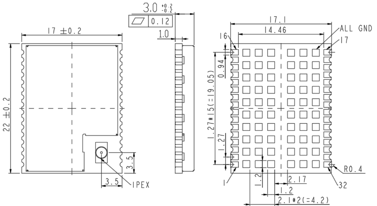
Figure 3. QD302 Dimension View / QD302 三视图
